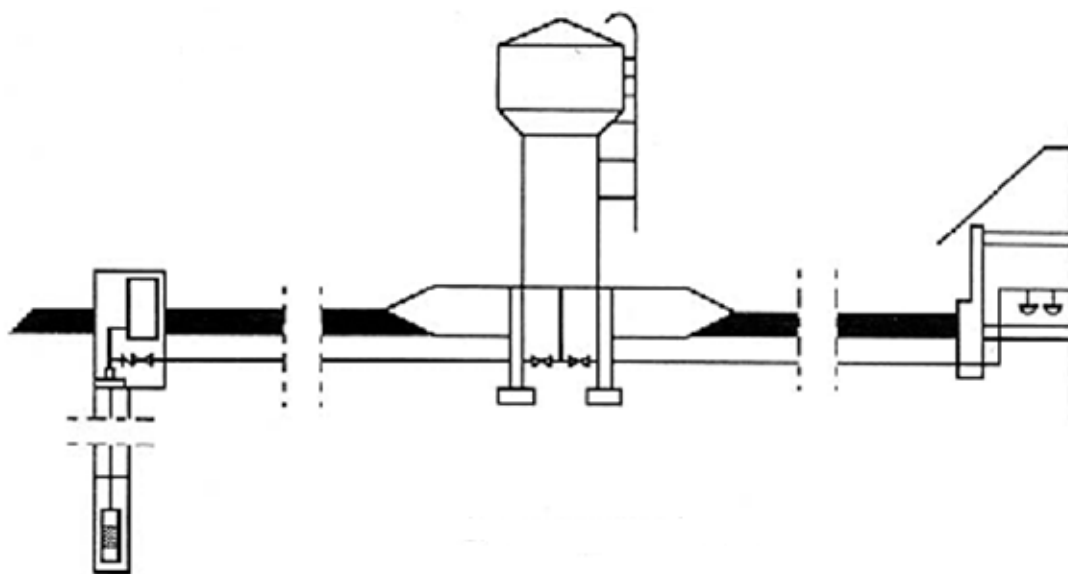
Рисунок 1-8. Схема водоснабжения населенного пункта при заборе воды из подземного источника
